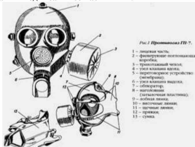
Рис.2 Противогаз ГП-7
