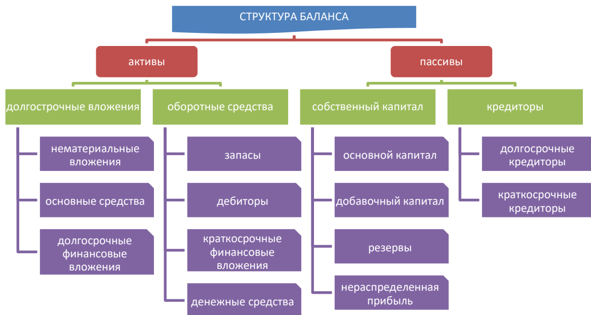
Рисунок 1 – Структура баланса
