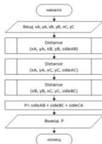
Рис.38 Основной алгоритм
