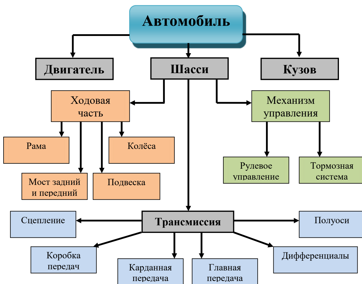
Рисунок 7 – Схема устройства автомобиля
