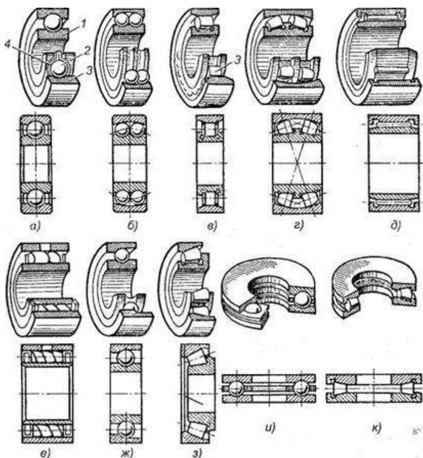
Рисунок 1 - Подшипники качения: а, б, в, г, е — радиальные подшипники; ж, з — радиально-упорные подшипники; и, к — упорные подшипники; 1 — внутреннее кольцо; 2 — тело качения; 3 — наружное кольцо; 4 — сепаратор.
