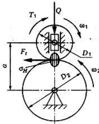
Рисунок 2 - Схема для расчета цилиндрической фрикционной передачи
