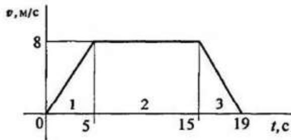
Рисунок 2 – График скорости
