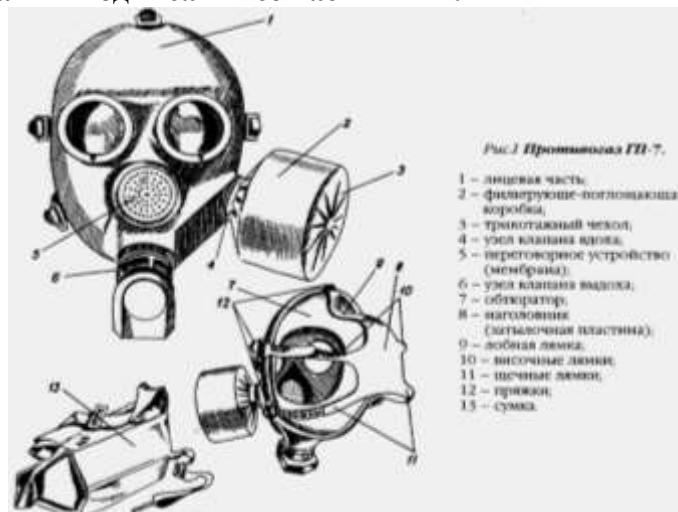
Рис.2 Противогаз ГП-7
