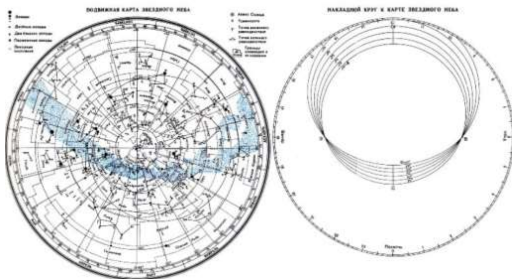
Подвижная карта звёздного неба изображена на рисунке.
