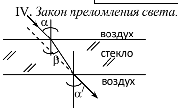
Рис. 13. Преломление светового луча.
