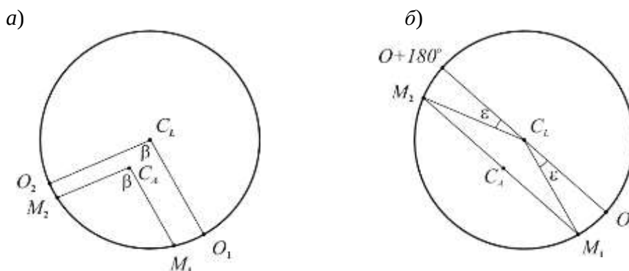
Рисунок 4. Эксцентриситет алидады: а – влияние на результат измерения угла; б – исключение влияния; C_L – центр лимба; C_A – ось вращения алидады.
