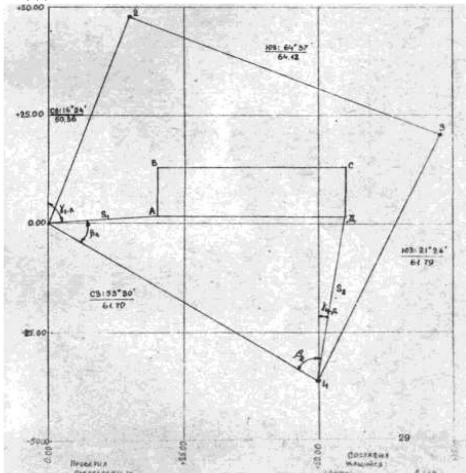
Рисунок 29 План теодолитного хода
