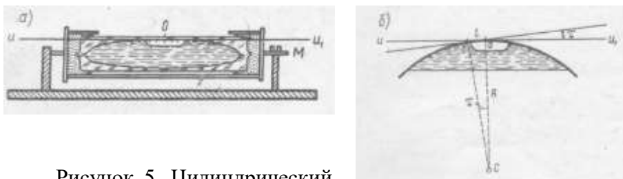
Рисунок 5. Цилиндрический уровень:
