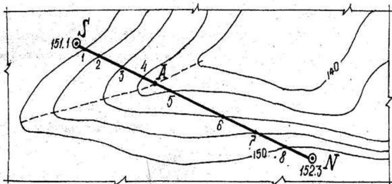
Рисунок 6.1 – Определение уклонов
