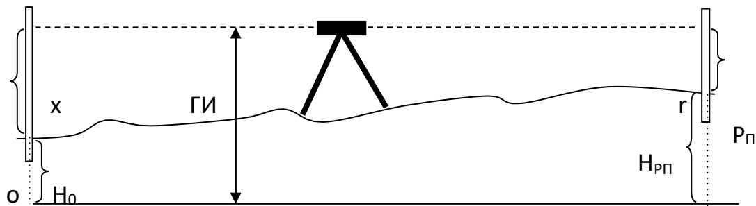
Рис. 19. Схема вынесения проектной отметки
