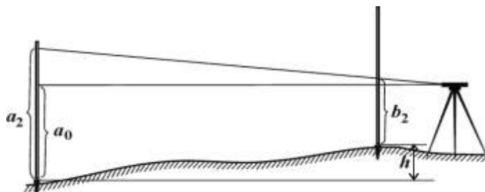
Рисунок 7. Поверка цилиндрического уровня. Измерения с неравными расстояниями до реек
