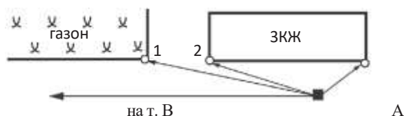
Рис. 16. Абрис тахеометрической съемки
