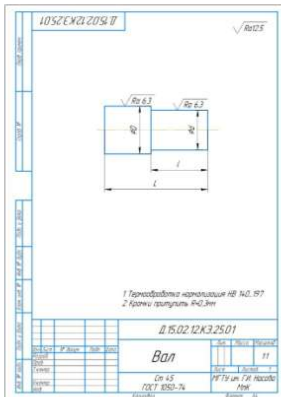
Рисунок 1- Чертёж детали
