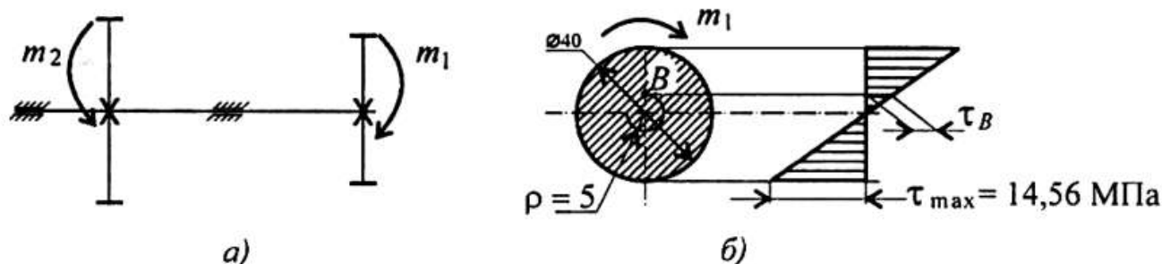
Рисунок 1 – Схема вала
