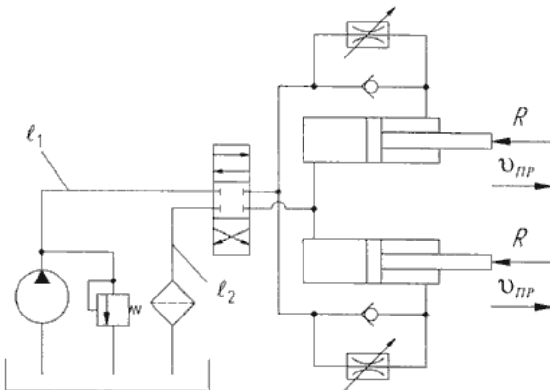
Рис.ХХ. Гидросхема привода поворота стрелы
