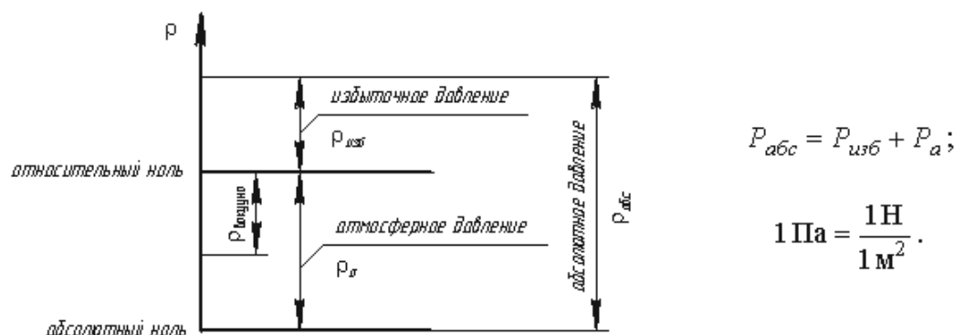
Рис. 1.5. Схема к определению давлений
