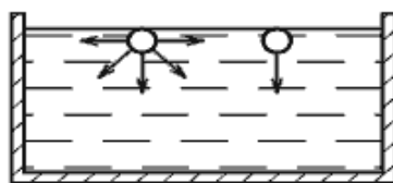
Рис. 1.6. Силы поверхностного натяжения
