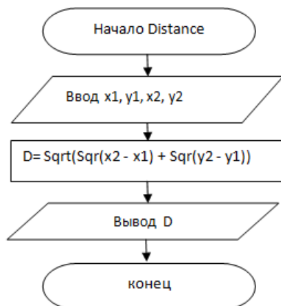
Рис.37 Вспомогательный алгоритм
