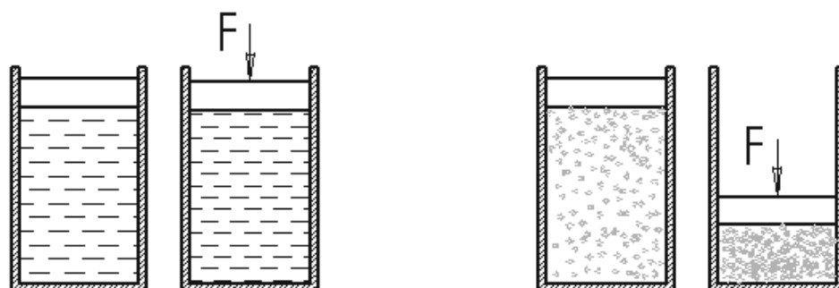
Рис. 1.3. Сжатие жидкостей и газов
