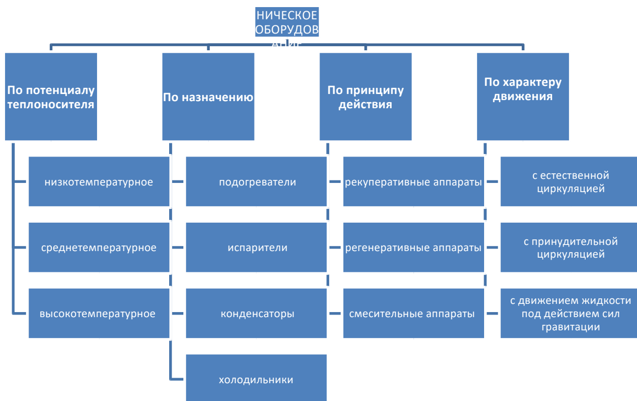
Рисунок 3 – Классификация теплотехнического оборудования
