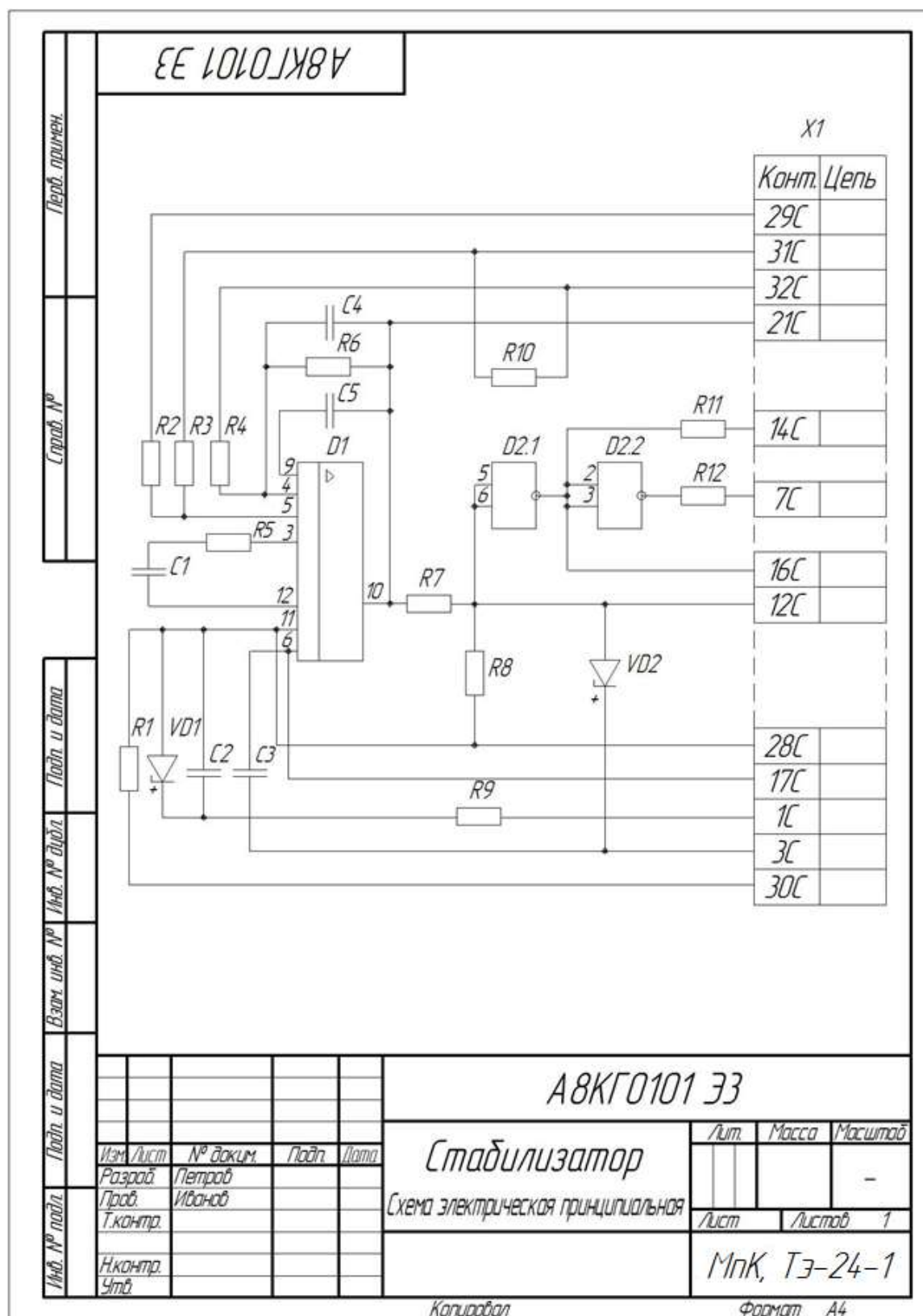
Рис.1. Пример выполнения и оформления схемы электрической принципиальной изделия «Стабилизатор»
