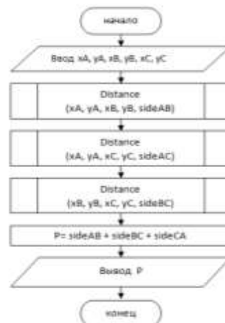
Рис.38 Основной алгоритм
