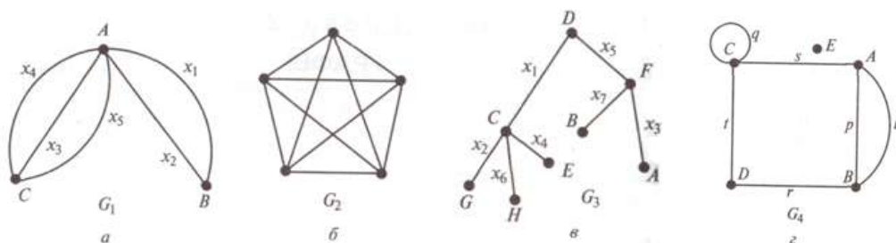
Рис. 1. Примеры графов: а – со смежными вершинами; б – полный; в – со смежными ребрами; г – с петлей
