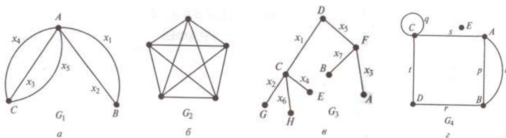
Рис. 1. Примеры графов: а – со смежными вершинами; б – полный; в – со смежными ребрами; г – с петлями
