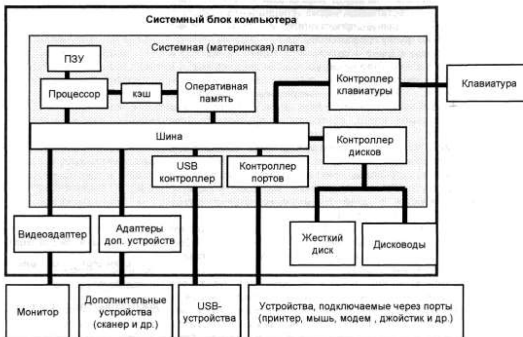
Рисунок 4 – Системный блок
