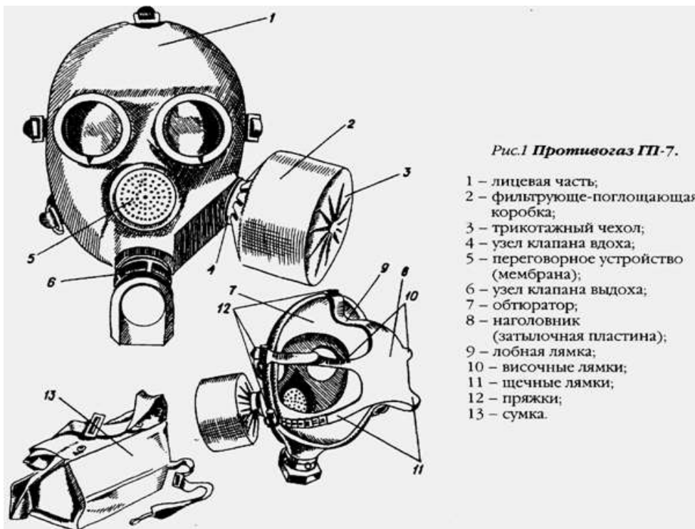
Рисунок 2- Противогаз ГП-7
