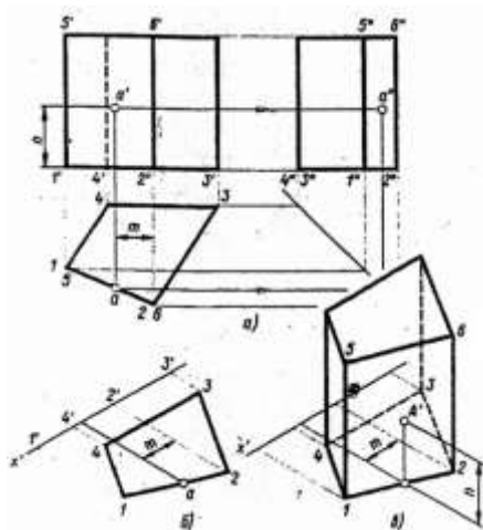
Рис.5 Проекция призмы
