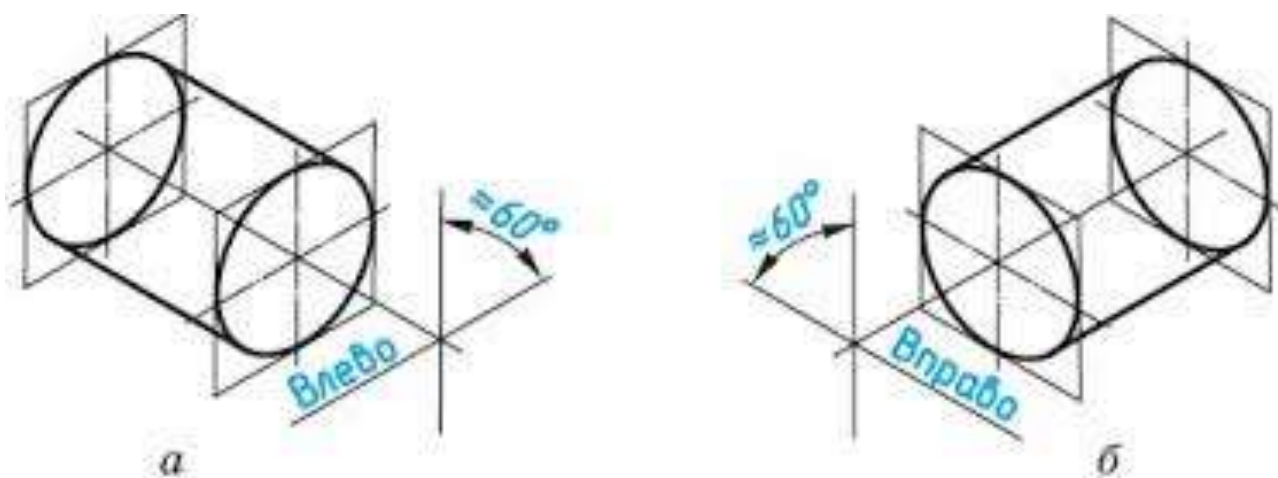
Рис15 Аксонометрия цилиндрической поверхности
