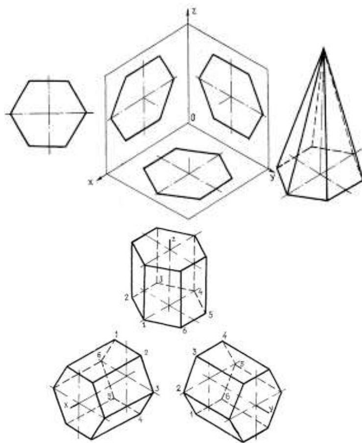
Рис.13 Аксонометрия многогранников
