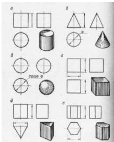
Рис.9 Проекции геометрических тел
