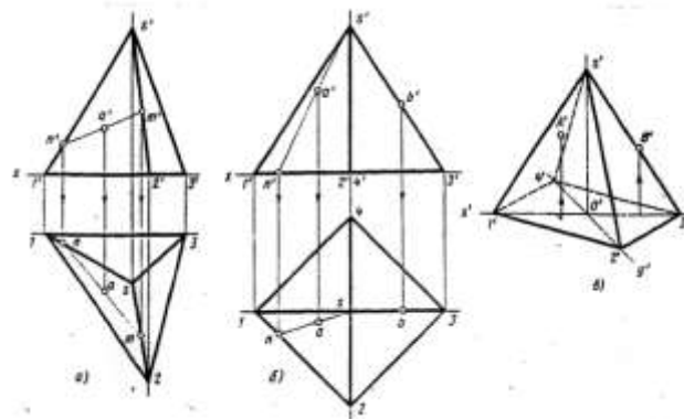
Рис. 6 Проекция пирамиды
