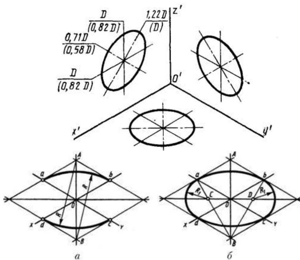
Рис.14 Аксонометрия окружности
