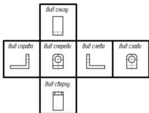
Рис.19 Основные виды
