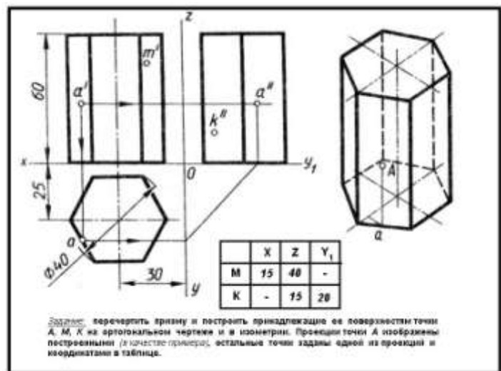
Рис.10 Проекции шестигранной правильной призмы
