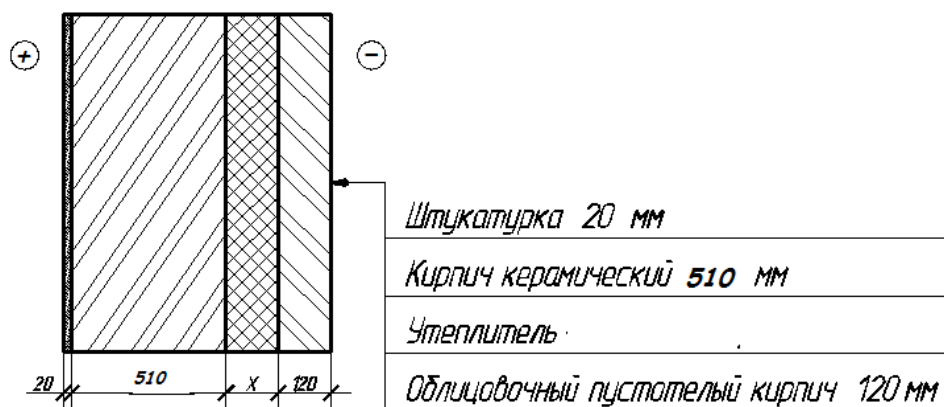
Рисунок 1 - Конструкция наружной стены
