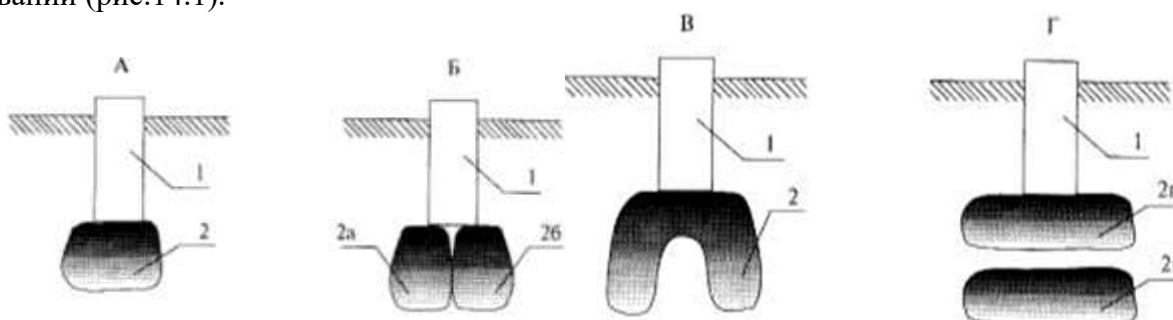
Рисунок 14.1 - Схемы устройства оснований из закрепленного грунта:
