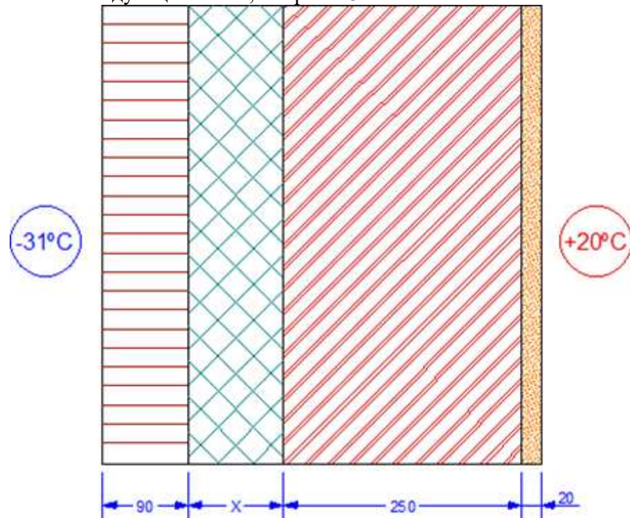
Рисунок 23.1 – Разрез стены
