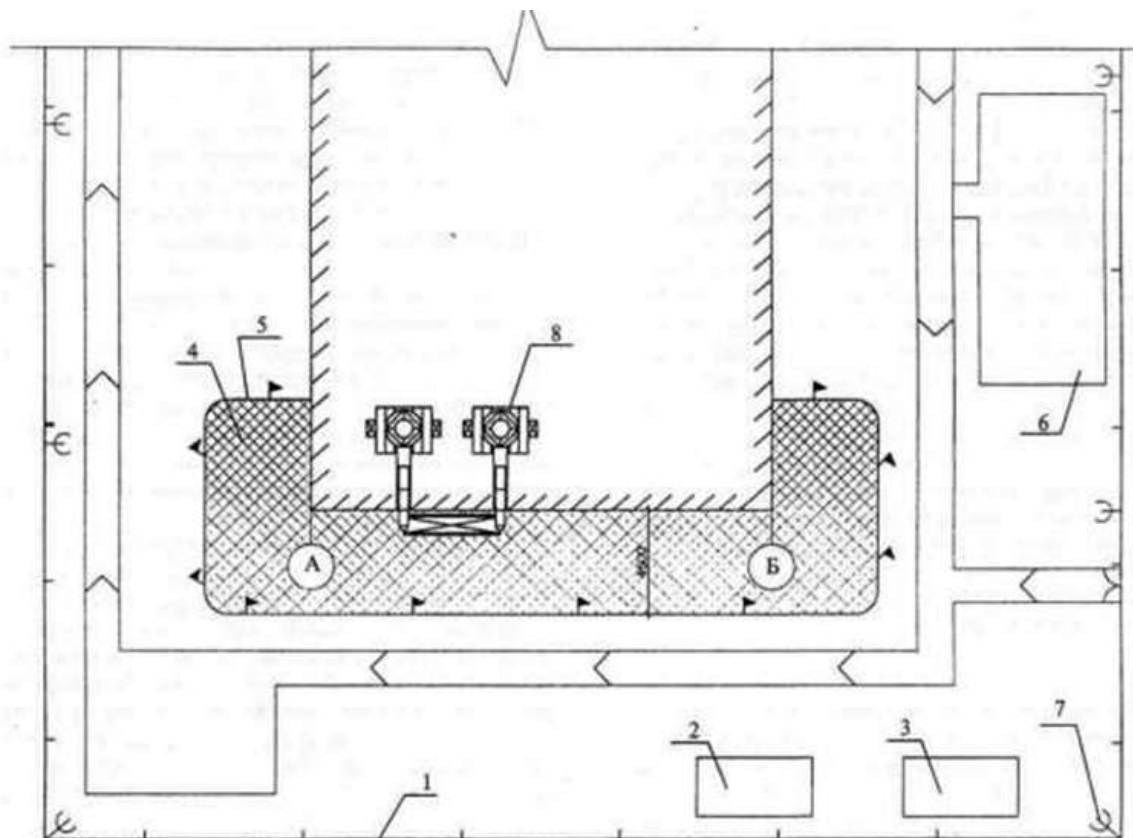
Рисунок 13.2 -. Схема организации строительной площадки
