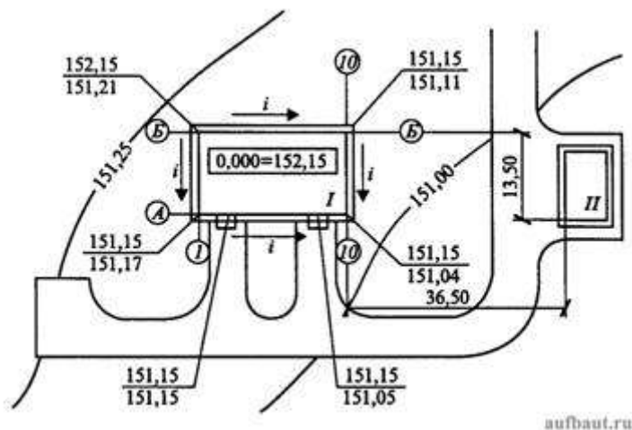
Рисунок 14. Пример выполнения вертикальной и горизонтальной привязок в учебной практической работе: I - проектируемое здание; II - существующее здание; i - направление стока поверхностных вод; А, Б, 1, 10 - обозначения осей
