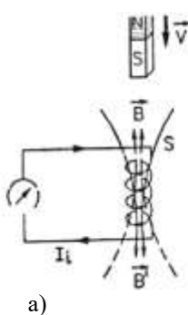
Рис. 3. Опыт, иллюстрирующий правило Ленца
