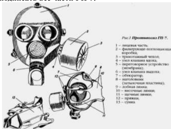
Рис.2 Противогаз ГП-7
