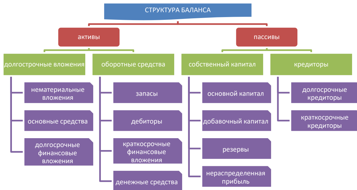
Рисунок 3 – Структура баланса
