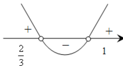
Рисунок 02. График функции
