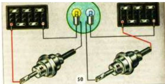
Рисунок 23 Проверка диода прямым (слева) и обратным (справа) включением его в цепь
