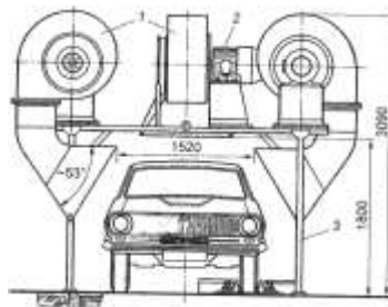
Назначение, устройство, тактико-технические данные воздуходувной установки ЦЛБ-111
