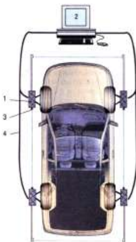
Рисунок 4 - Компьютерный стенд для измерения углов установки колес: 1 – датчики; 2 – компьютер; 3 – инфракрасные датчики связи; 4 – соединительные провода
