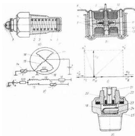
Рисунок 1. Датчик температуры: а) датчик ТМ - 100 с терморезистором;
