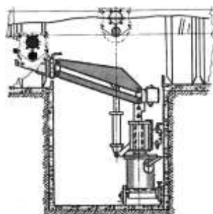
Универсальный стелд для демонтажа коробок передач грузовых автомобилей на осмотровых канавах
