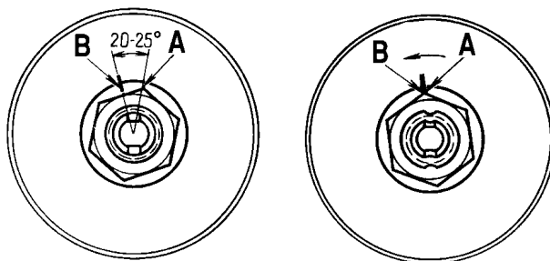
Рисунок 6 - Схема затяжки гайки ступицы
