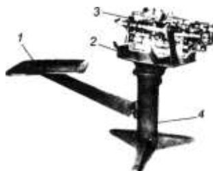
Универсальный стелд для разборки и сборки коробок передач грузовых автомобилей: 1 — подставка; 2 — ложемент-манипулятор; 3 — коробка передач; 4 — стойка
