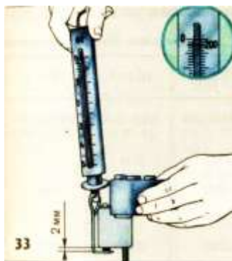
Рисунок 9. Проверка пружины щеток с помощью динамометра
