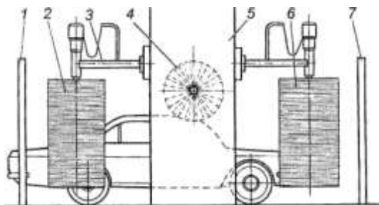
Щеточная установка для мойки легковых автомобилей: 1 — рамка для смачивания; 2 — входной блок вертикальных щеток; 3 — каретка с консолями; 4 — горизонтальная щетка; 5 — рама; 6 — выходной блок вертикальных щеток; 7 — рамка для ополаскивания автомобиля
