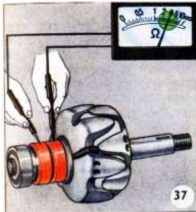
Рисунок 12. Измерение сопротивления обмотки возбуждения омметром
