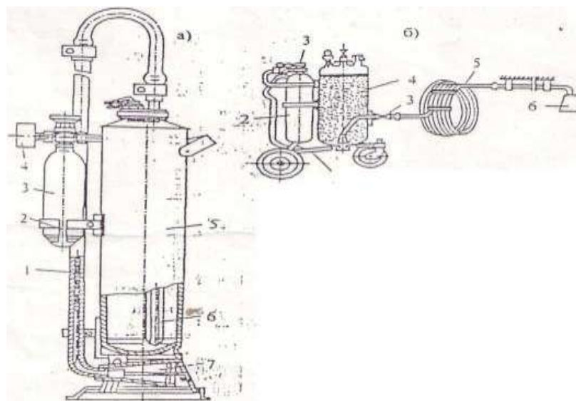
Рис.4 а) порошковый огнетушитель ОПС-10: 1 - удлинитель, 2 - кронштейн, 3 - баллон, 4 - манометр, 5 - корпус, 6 - сифонная трубка, 7 - насадка;
