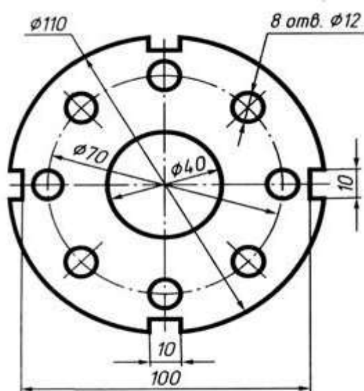
Прокладка
