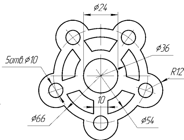
Прокладка
