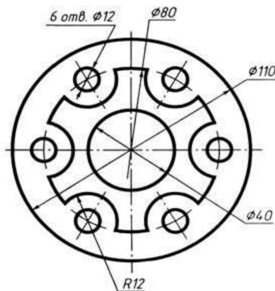
Прокладка
