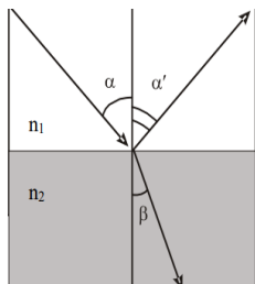
Рис. 2. Законы отражения и преломления света
