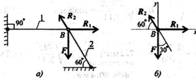
Рисунок 1 – Груз на стержне
