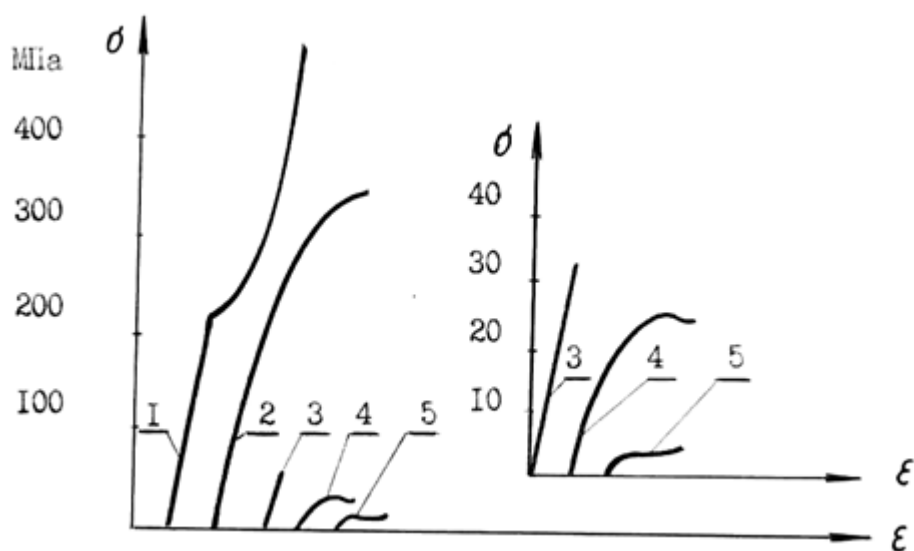
Рисунок 1 - Диаграммы сжатия:
