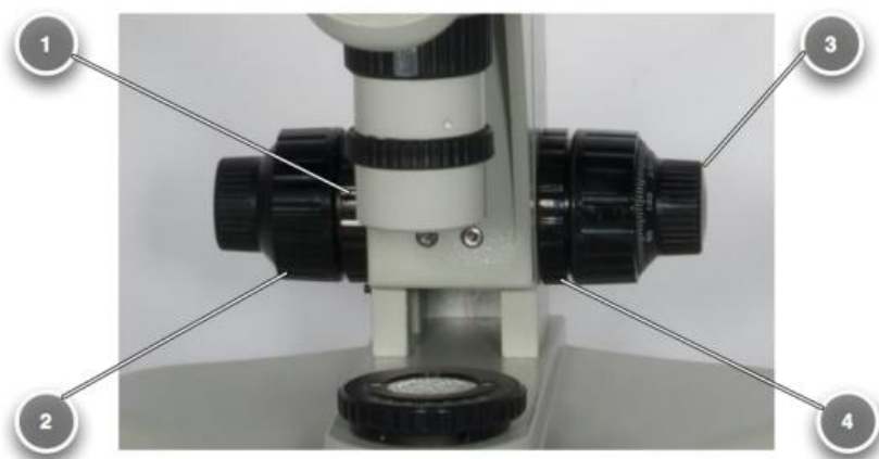
Общий вид фокусирующего механизма
