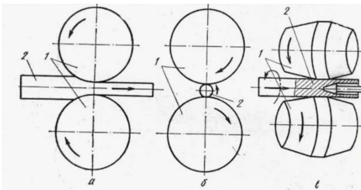
а – продольная прокатка; б – поперечная прокатка; в – косая прокатка
