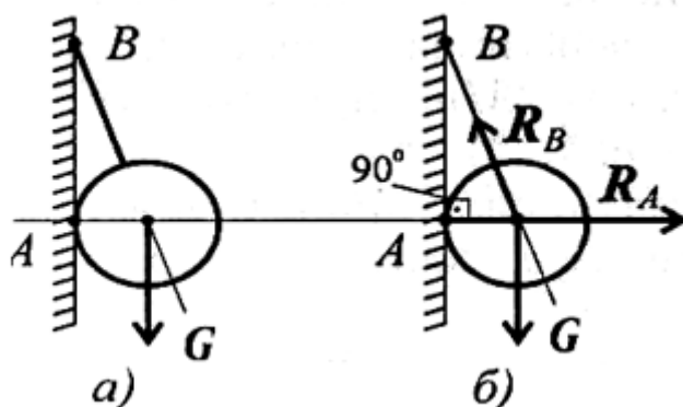
Рисунок 2 - Определение реакции нити и гладкой опоры а) шар на нити; б) реакции
