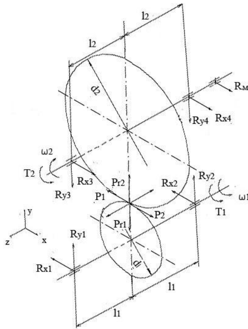
Рисунок 2 - Схема нагружения валов
