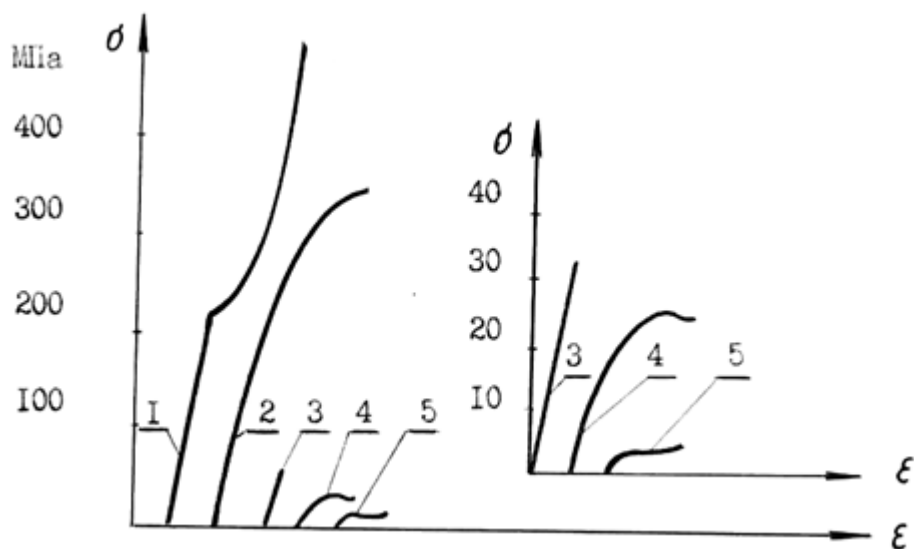
Рисунок 1 - Диаграммы сжатия:
