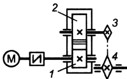
1 – быстроходный вал; 2 – тихоходный вал; 3 – ведущая звездочка; 1 – ведомая звездочка
