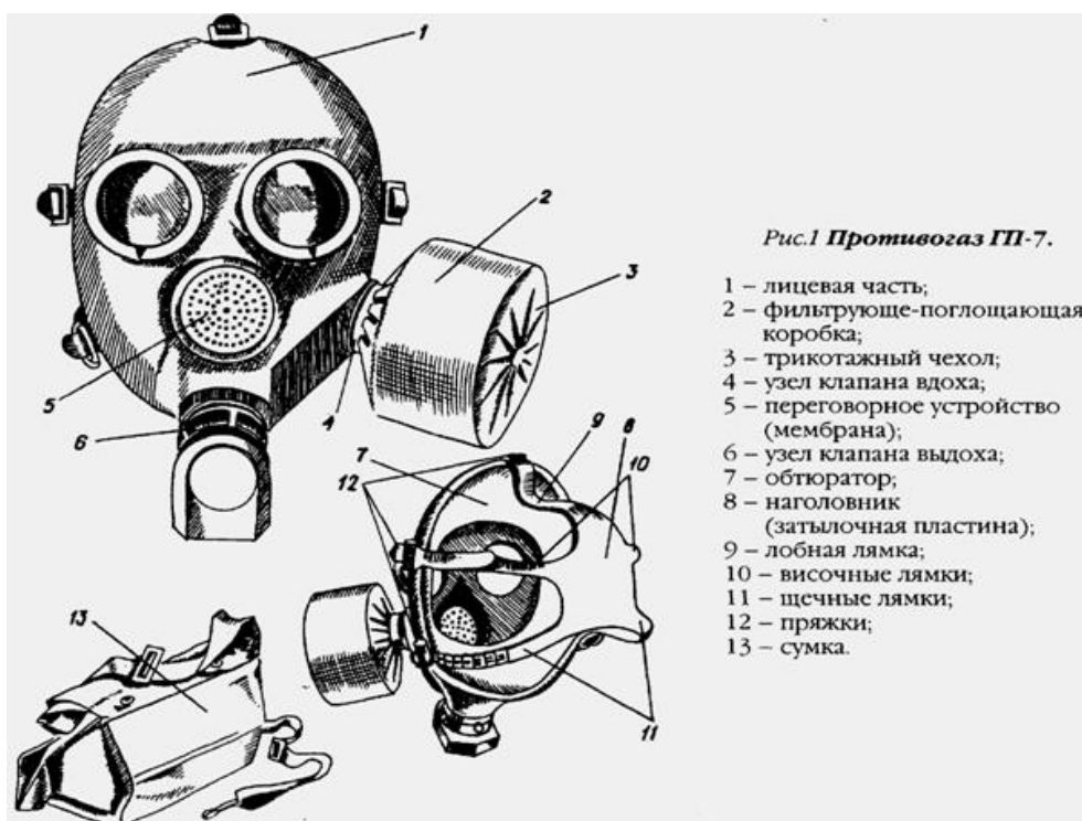
Рисунок 2- Противогаз ГП-7
