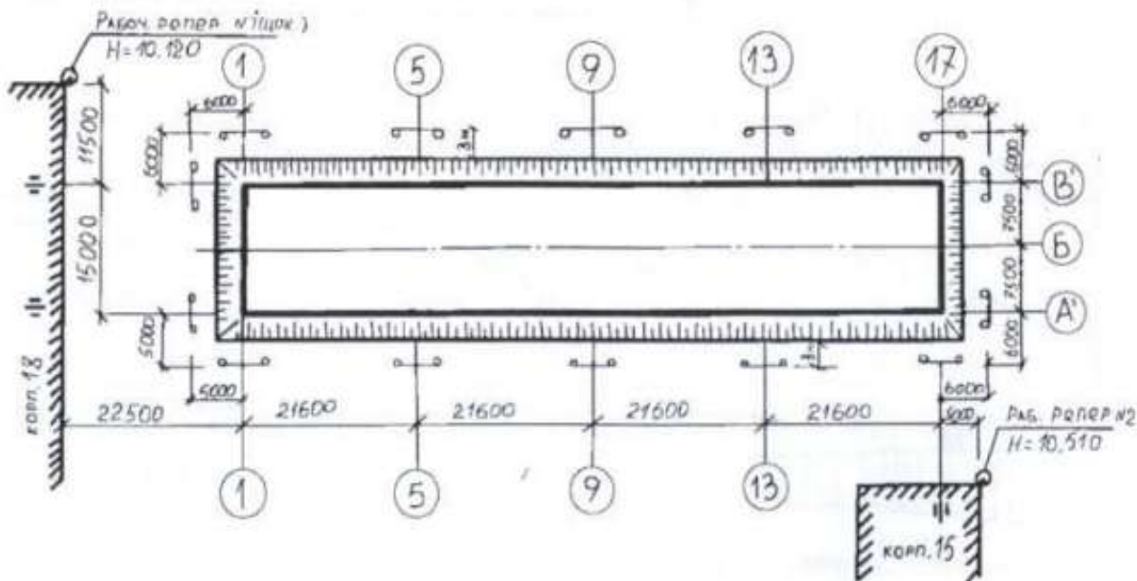
Рисунок 26 Исполнительная схема разбивки осей здания.
