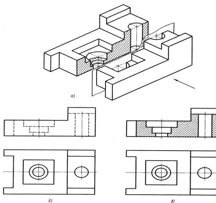
Рисунок 41 - Разрез
