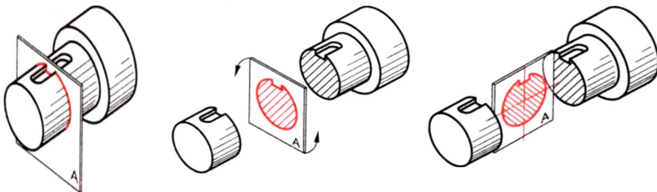
Рисунок 38 - Сечение
