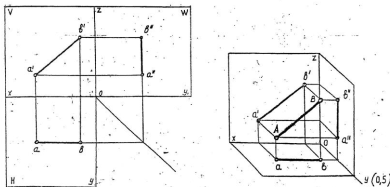
Рисунок 14 - Проекция прямой
