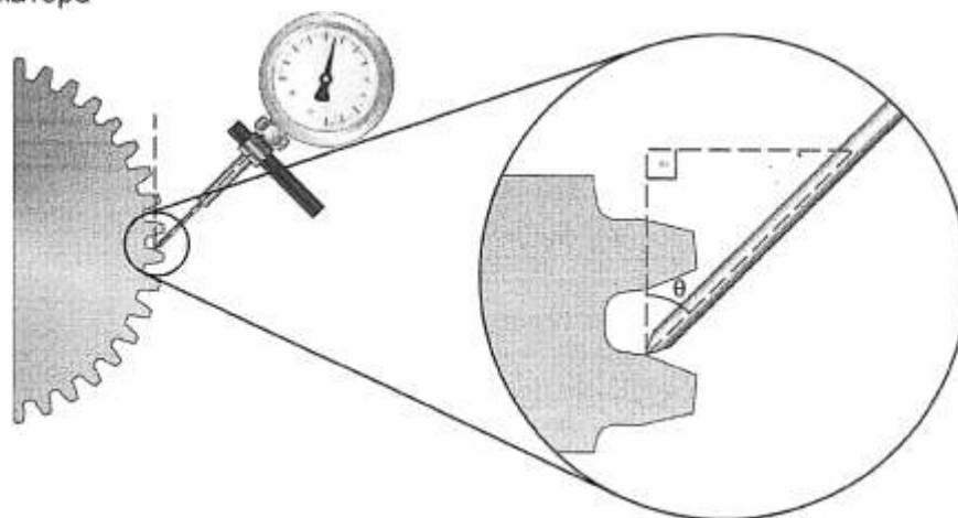
Погрешность измерения бокового зазора в силу эффекта косинусной ошибки.
