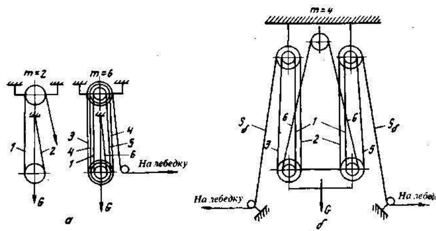
Рисунок 1.6 - Схемы полиспастов
