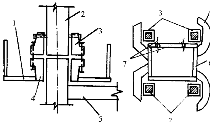
Рис. 4. Одиночный (а) и групповой (б) кондукторы для временного закрепления колонн:
