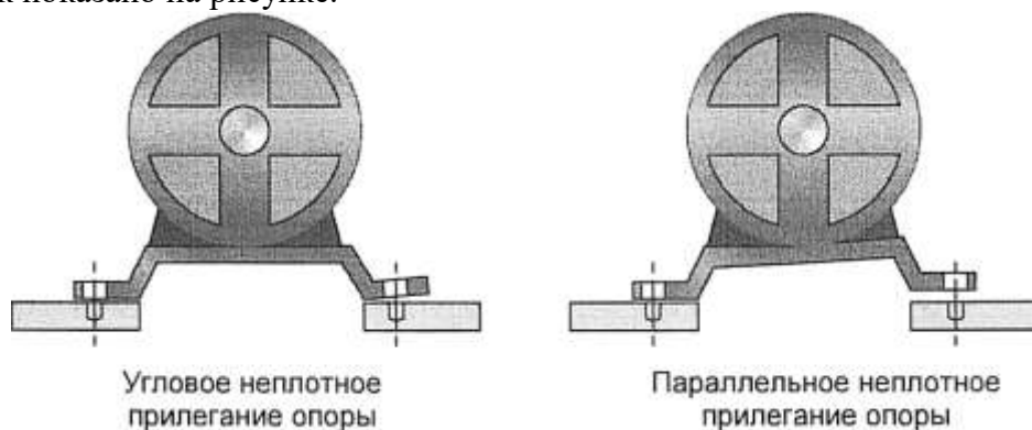
Рисунок. Дефект опоры электродвигателя - параллельное и угловое неплотное прилегание опоры.
