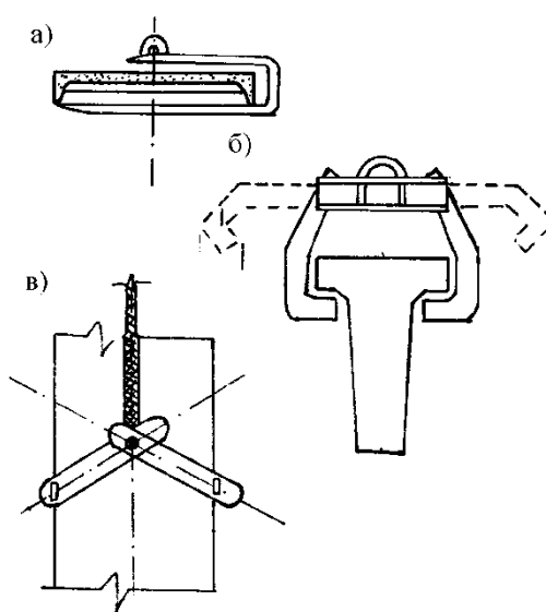
Рис. 3. Беспетлевые захваты
