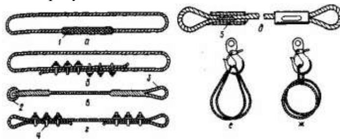
Рисунок 1.4 - Универсальные стропы
