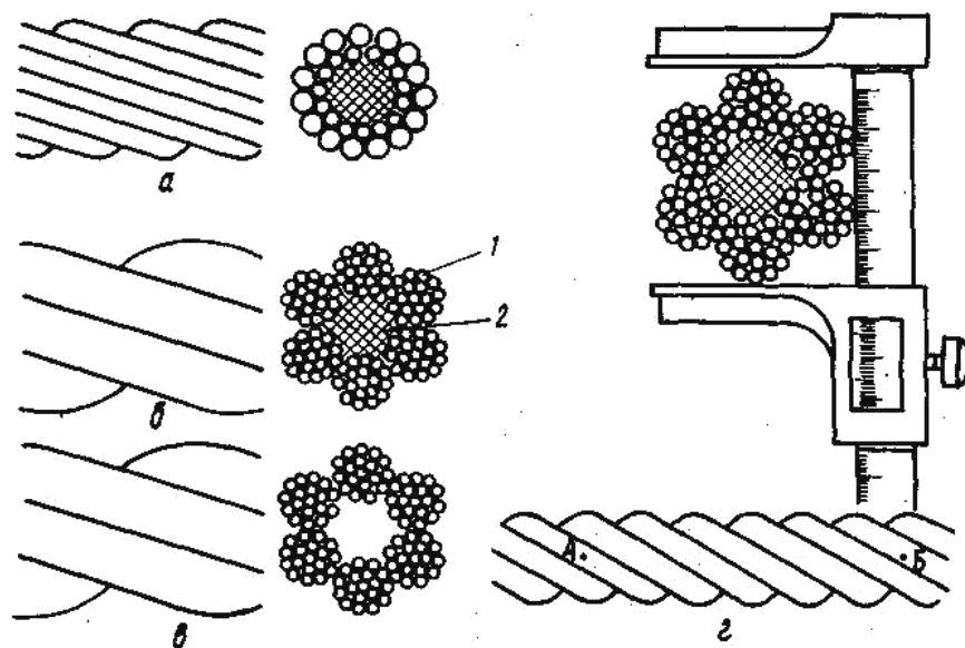
Рисунок 1.1 - Стальные канаты
