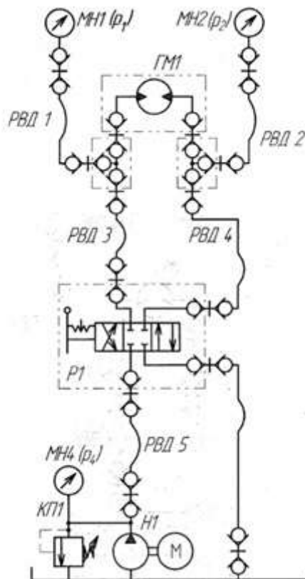
Рисунок 2 - Гидросхема
