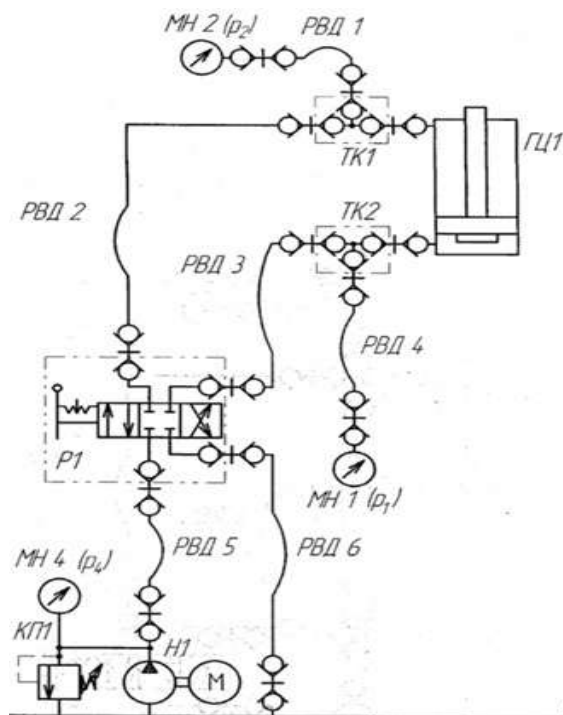
Рисунок 1- Гидросхема
