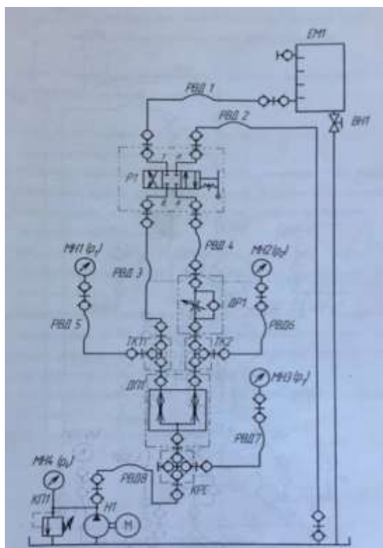
Рисунок 1 - Гидросхема
