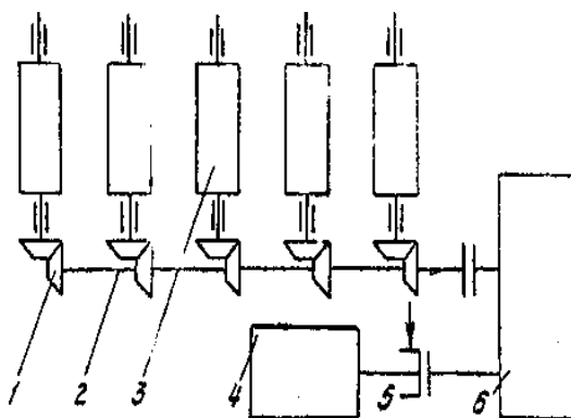
Рисунок 1- Привод рольганга
