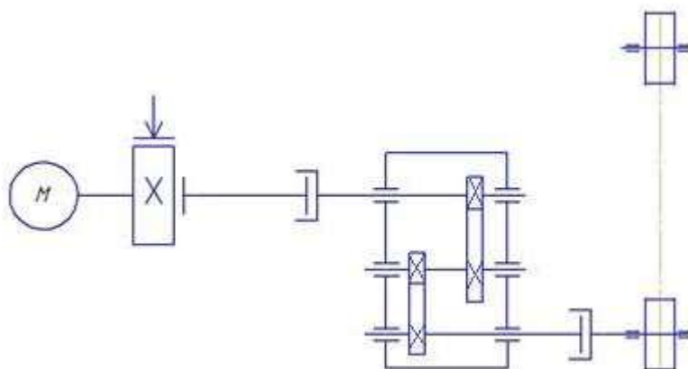
Рисунок 1 – Кинематическая схема привода механизма перемещения мостового крана
