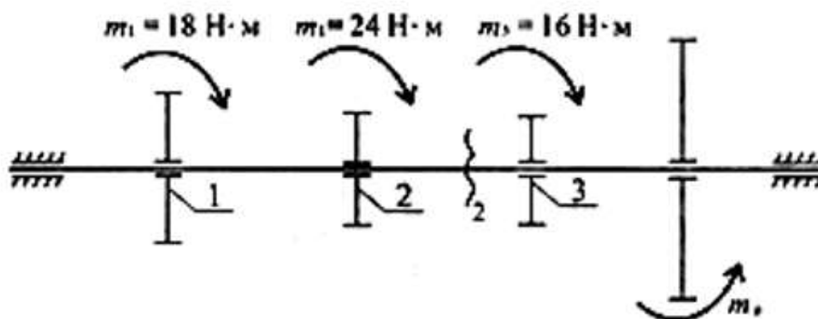
Рисунок 2 – Схема вала
