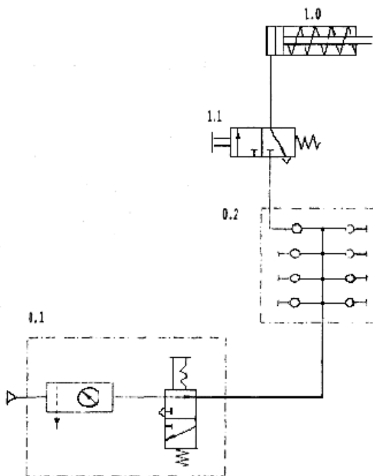
Рисунок 1 - Принципиальная схема
