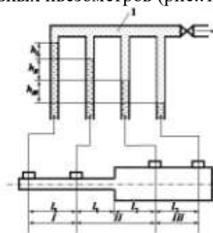
Рисунок -1. Измерение разности напоров на местном сопротивлении. 1-блок дифференциальных пьезометров; l_I, l_{II} –длины участков I и III; l_1, l_2 –длины участка II непосредственно перед и после внезапного расширения; h_I, h_{II}, h_{III} – потери напоров на участках I, II, III.
