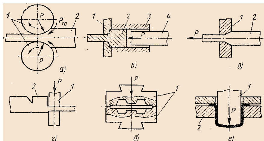
Рис. 1. Схемы основных видов обработки металлов давлением
