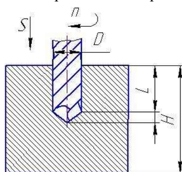
Рисунок 1 – Эскиз обработки
