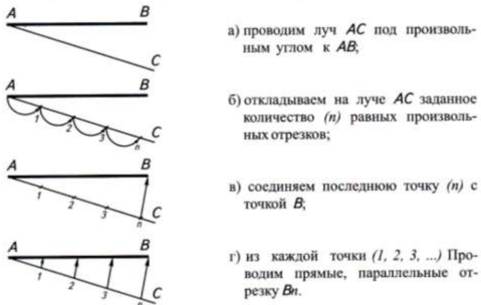
Рис 6 Деление отрезка равные отрезки
