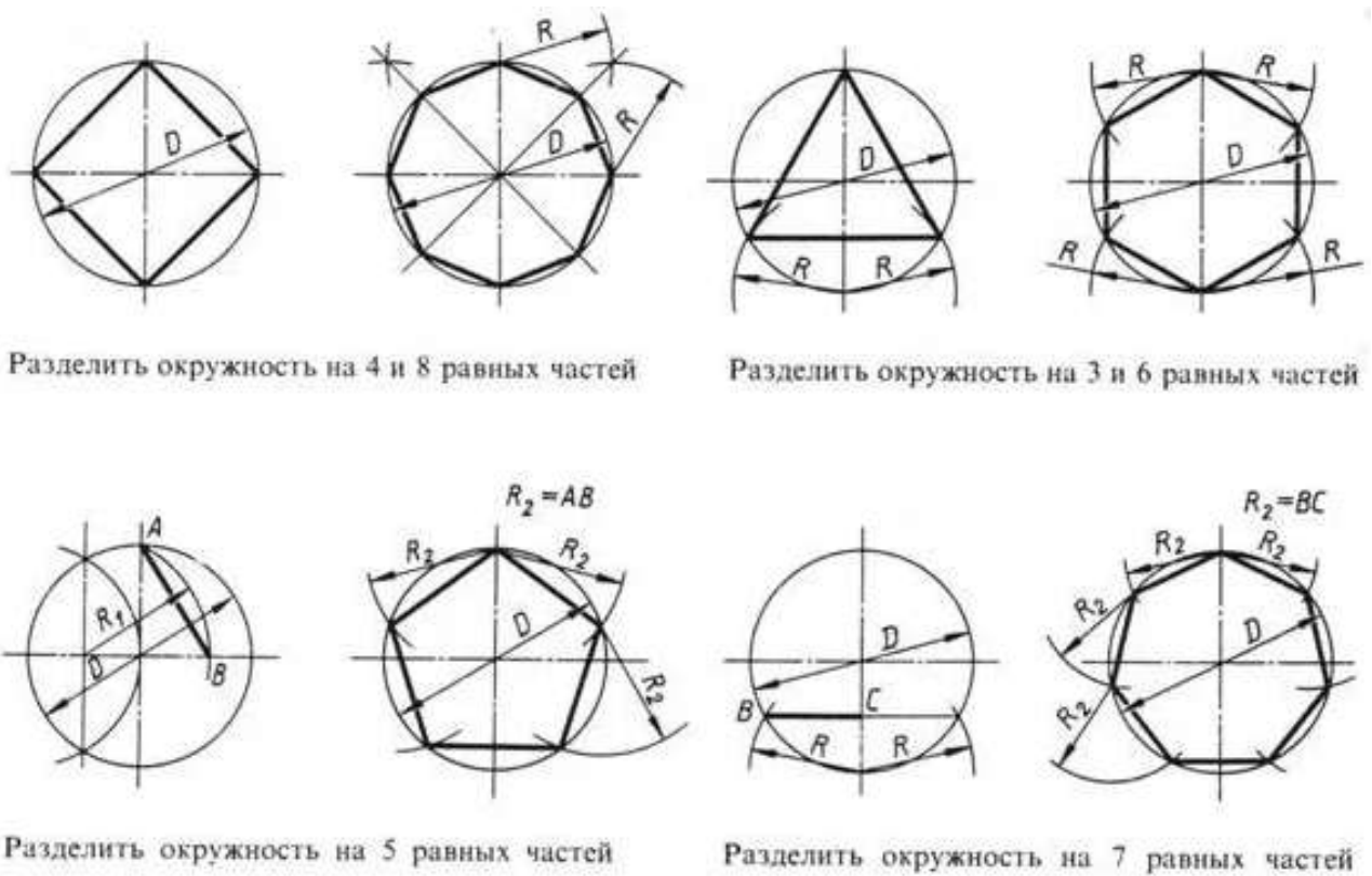
Рис.5 Деление окружности на равные части
