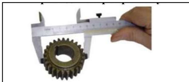
Рис.58 Определение диаметра вершин зубьев колеса
