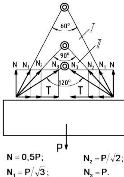
Рисунок 20.1 Схема распределения нагрузок на ветви стропа: I – рекомендуемая зона захвата груза; II – нерекомендуемая зона захвата груза
