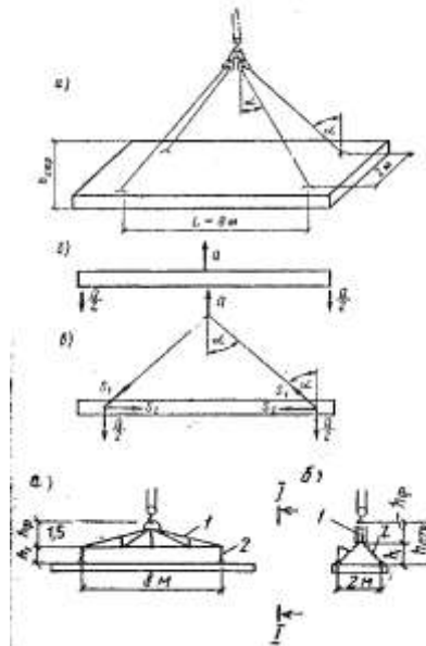
Рисунок 20. 3 Строповка конструкций:
