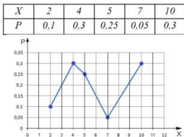
Рисунок 1 – Многоугольник распределения для данного ряда распределения ДСВ
