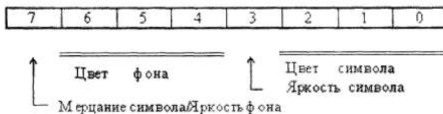
Рис. 2.1.- Структура байта атрибутов
