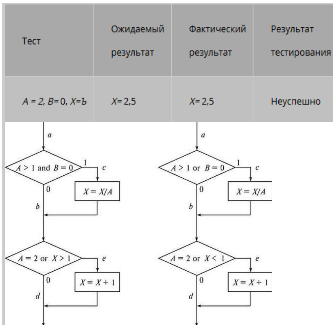
Рис. Л5.1. Пример алгоритма программы: a — правильный; b — с ошибкой
