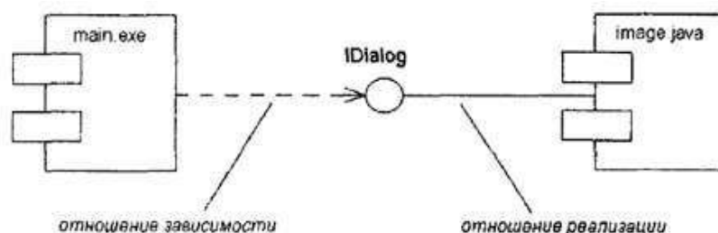
Рис. 4. Фрагмент диаграммы компонентов с отношением зависимости
