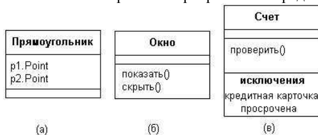
Рис.2. Примеры графического изображения классов на диаграмме
