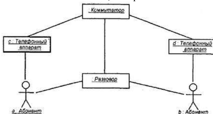
Рис. 8. Начальный фрагмент диаграммы кооперации для примера моделирования обычного телефонного разговора
