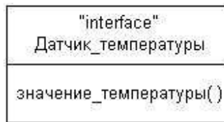
Рис. 10. Пример графического изображения интерфейса на диаграмме классов
