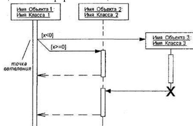
Рис. 12. Графическое изображение различных видов сообщений между объектами на
