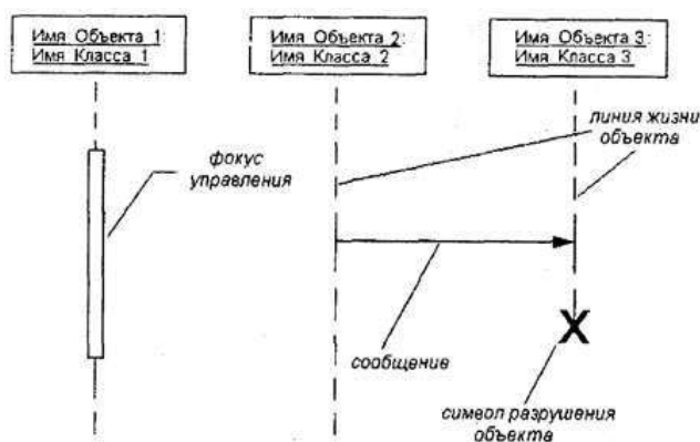
Рис. 9. Различные графические примитивы диаграммы последовательности
