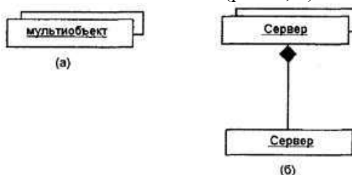
Рис. 5. Графическое изображение мультиобъектов на диаграмме кооперации
