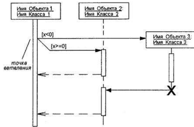
Рис. 13 Графическое изображение бинарного ветвления потока управления на диаграмме последовательности
