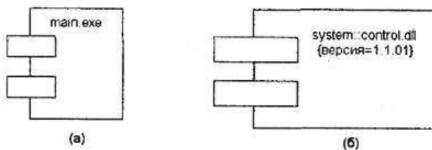
Рис. 1. Графическое изображение компонента в языке UML
