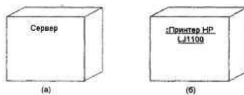
Рис.1. Графическое изображение узла на диаграмме развертывания
