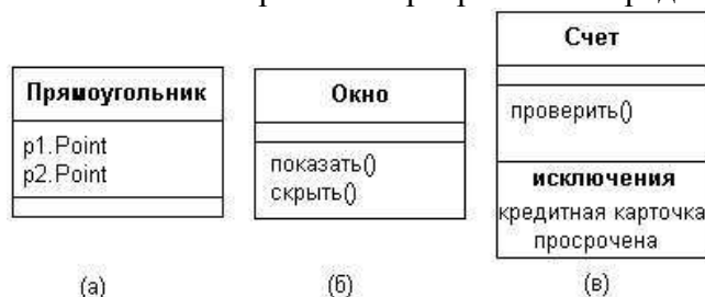
Рис.2. Примеры графического изображения классов на диаграмме
