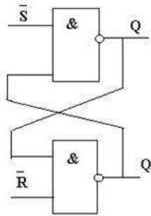
Рис. Асинхронный триггер на логических элементах И-НЕ
